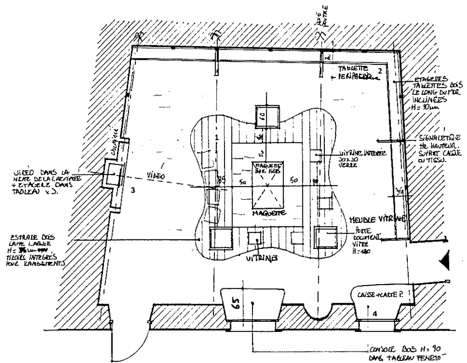
PLAN D'AMENAGEMENT ech 1/50°
